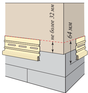
Рис. 17. Накладка облицовки на цоколь
