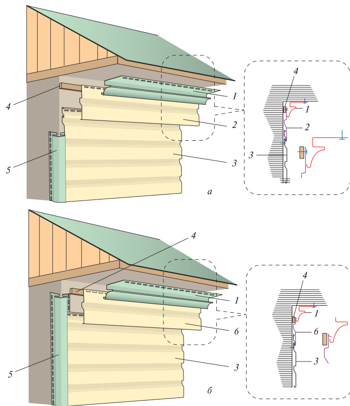
Рис. 39. Схема монтажа сайдинга прикрываемым молдингом Döcke: а – на крепежах; б – на зацепах; 1 – молдинг Döcke; 2 – подкарнизный сайдинг с дополнительными гвоздевыми отверстиями; 3 – рядовой сайдинг; 4 – выравнивающая рейка; 5 – угловой сайдинг; 6 – подкарнизный сайдинг с «зацепами»
