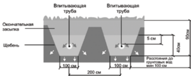
Рис. 5 Поперечное сечение впитывающей траншеи (площадки)
