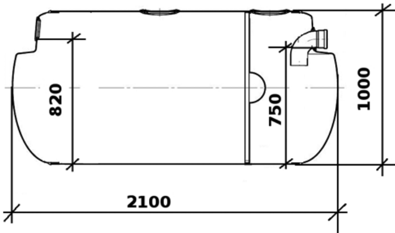
Рис. 1 Схема септика FloTenk - STA
