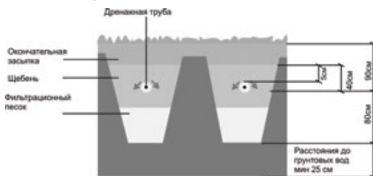
Рис. 7 Поперечное сечение поля фильтрации
