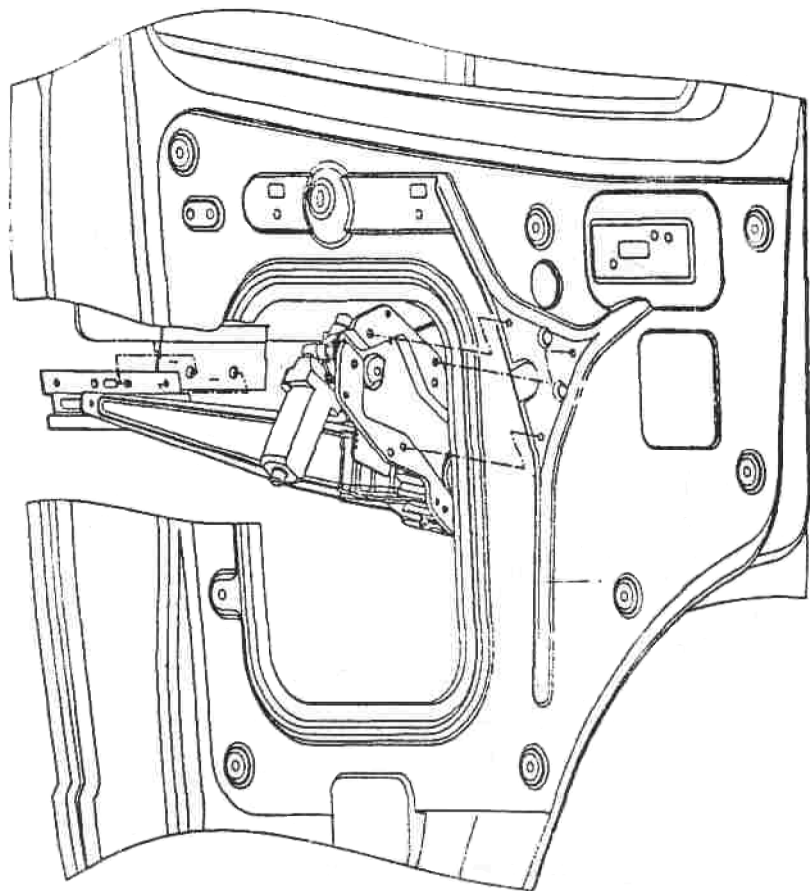
Рис. 2. Схема установки электростеклоподъемника в переднюю левую дверь
