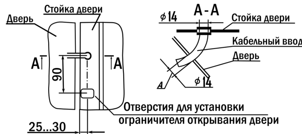
Рис. 1. Установка кабельного ввода
